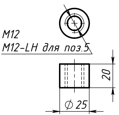
Поз.5 и Поз.6 (Гайка)
