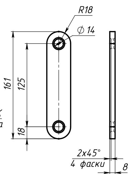
Поз.9 (Серьга)
