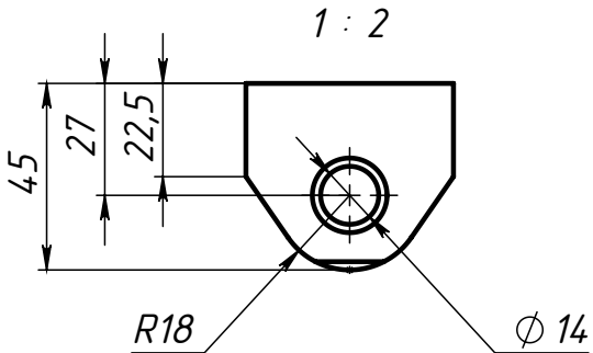
Поз.1 (Проушина)
