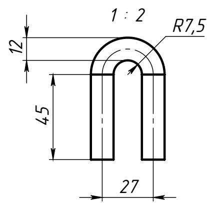
Поз.2 (Ушко)
